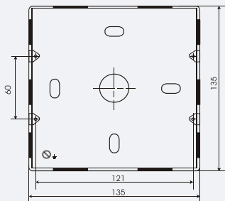
8 & 10 Module
