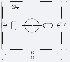
1, 2 & 3 Module
