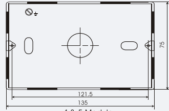
4 & 5 Module
