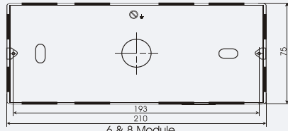
6 & 8 Module
