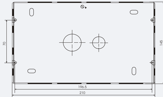
16 Module
