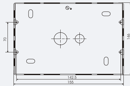
12 Module
